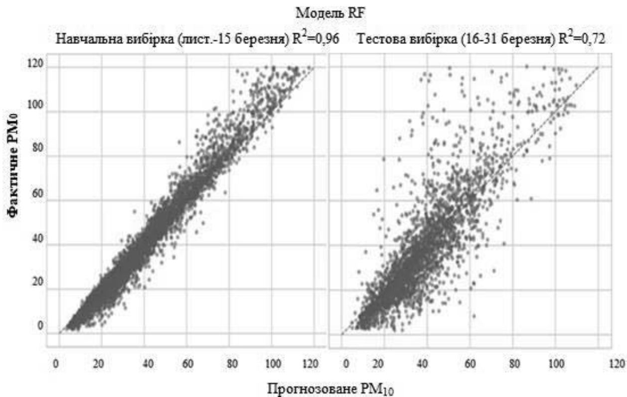
Рисунок 5 - Оцінка точності моделі Random Forest
