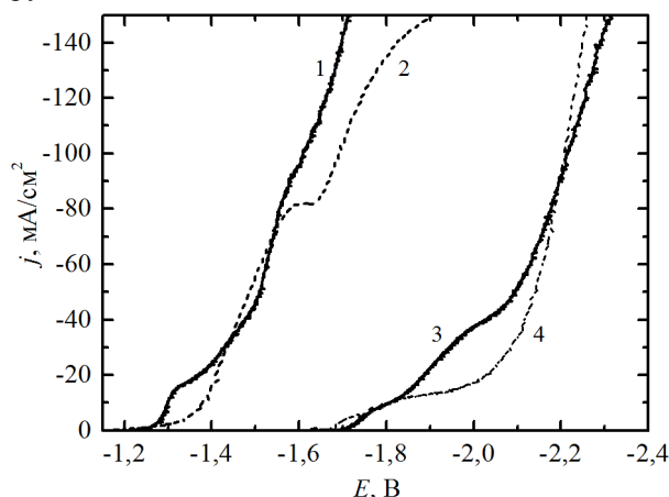
Електроліт: 1 – хлоридний, 2 – амікатний, 3 – лужний з добавками Grovision Base+Britghtener, 4 – лужний з добавкою Колцинк АЦФ
