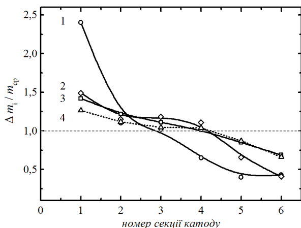
Електроліт: 1 – хлоридний, 2 – амікатний, 3 – лужний з добавками Grovision Base + Brightener, 4 – лужний з добавкою Колцинк АЦФ
